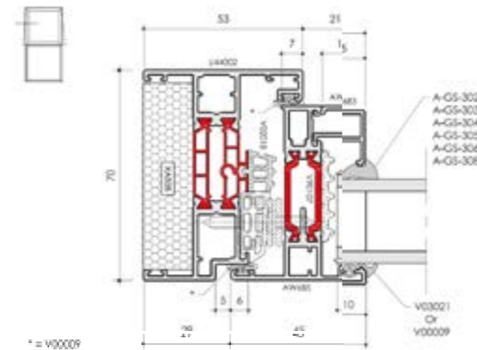
■ Jamb Section
